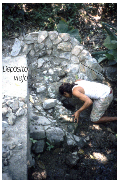
Pared para prevenir la contaminación de la toma de los vecinos con agua superficial
